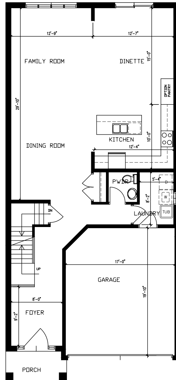
GROUND FLOOR PLAN B 1130 S.F. PLAN B : 2617 S.F.
